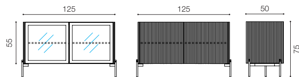
Madia 120 ante battenti vetro o legno / Sideboard 120 hinged glass or glass doors
